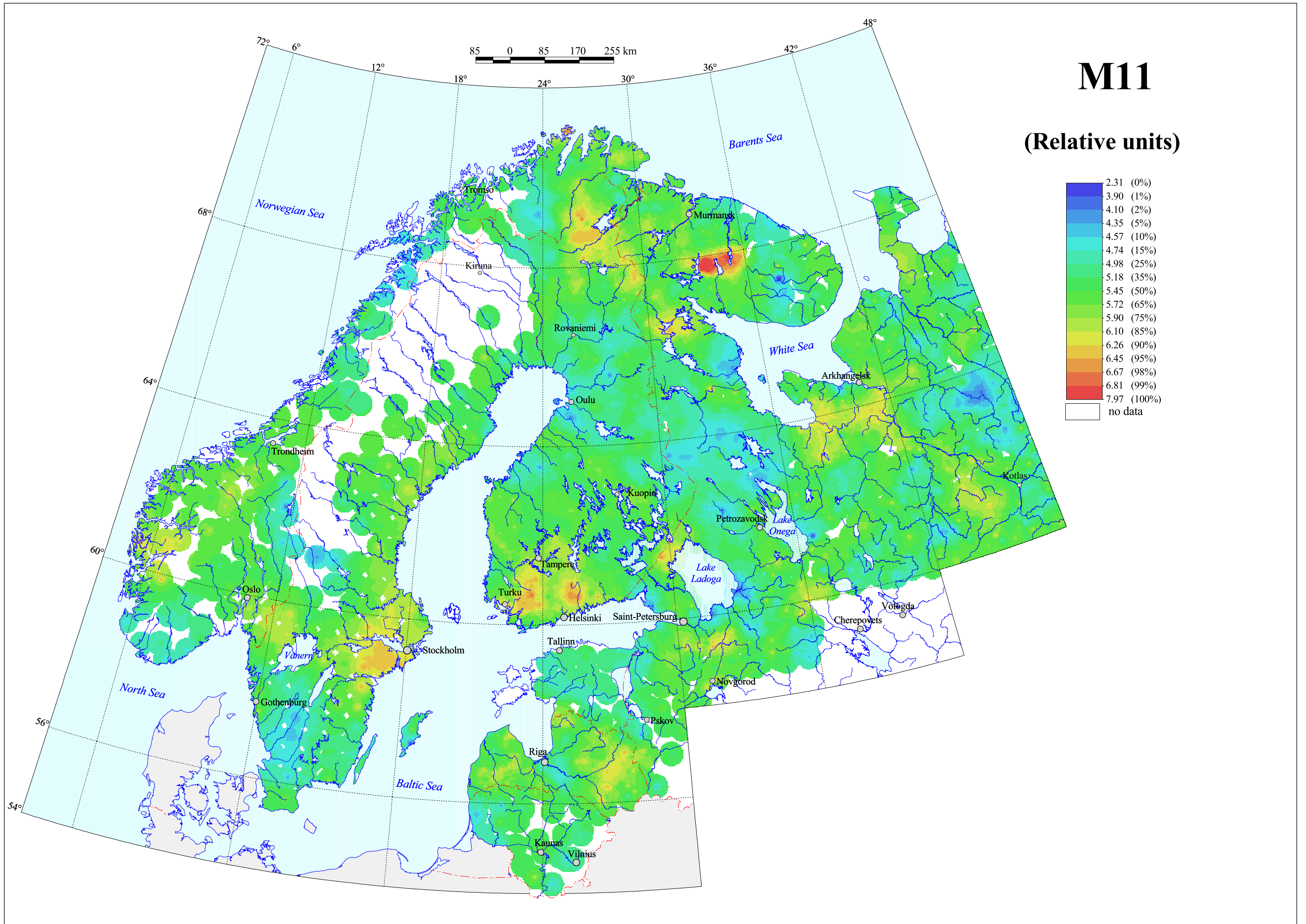
M11 (Al, Ba) in C-horizon, Grain Size <2 mm, Aqua regia Extraction
